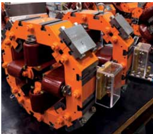
O engenheiro Rafael Seraphim realiza teste do sistema de vácuo das câmaras que conduzirão os elétrons. Ao lado, magnetos quadrupolos, um dos componentes do anel de armazenamento
